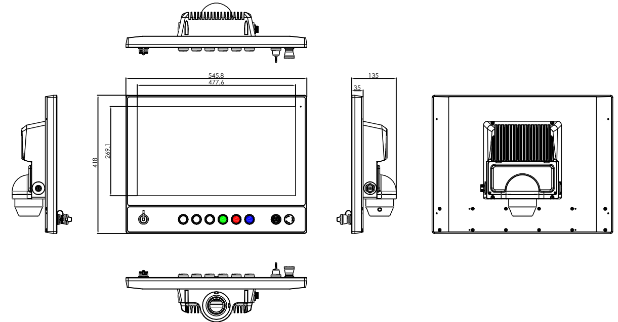
ABOS-921DP Stand
